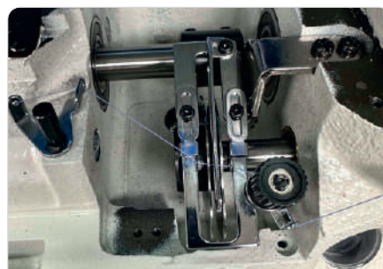
Вал нити снаружи
