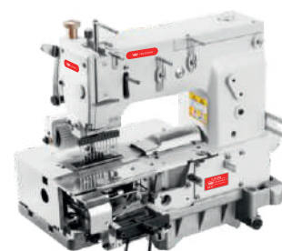
V-1412PQ 12-игольная, средняя нить эластичная
