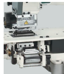
VSP: Устройство для вытягивания нижней эластичной нити
