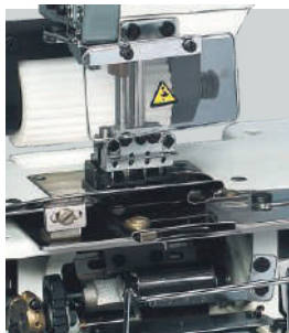
VWL: Роликовое устройство подачи переднего эластичного ремня
