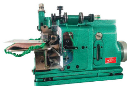
V-209 Лого машина с рукоятью
